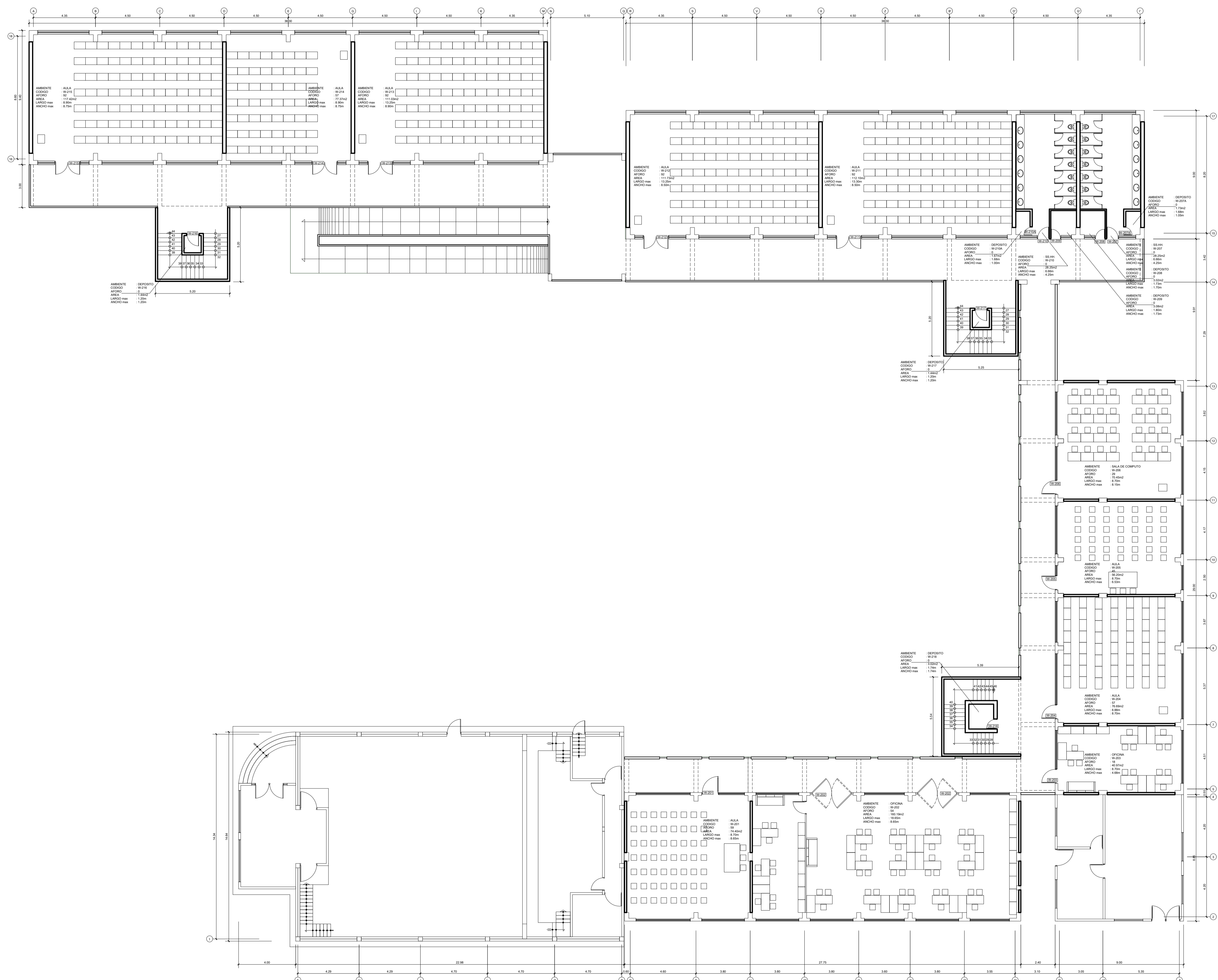
SEGUNDA PLANTA AREA TECHADA = 1690.92m 2 AFORO = 687 ESCALA 1:100
